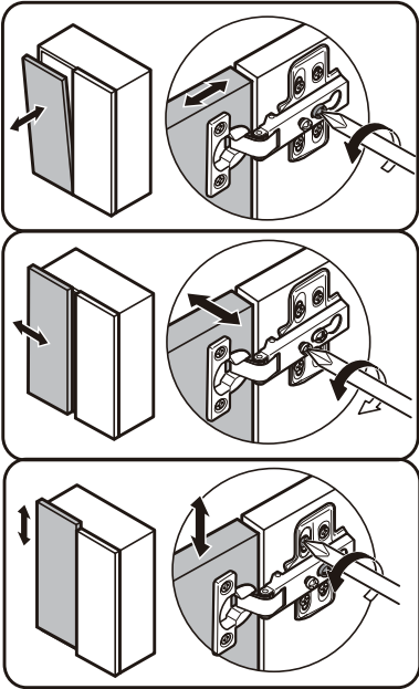
門片密合度調整
